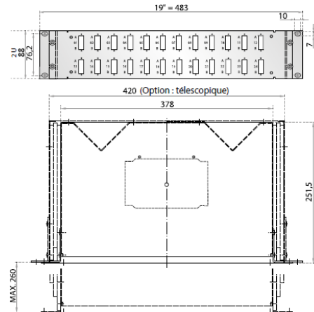
DIMENSIONS 2 U
