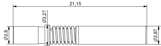
Buchse
