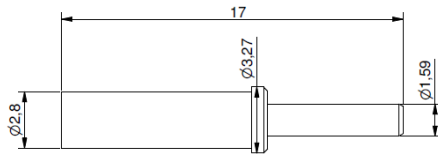
Stecker
